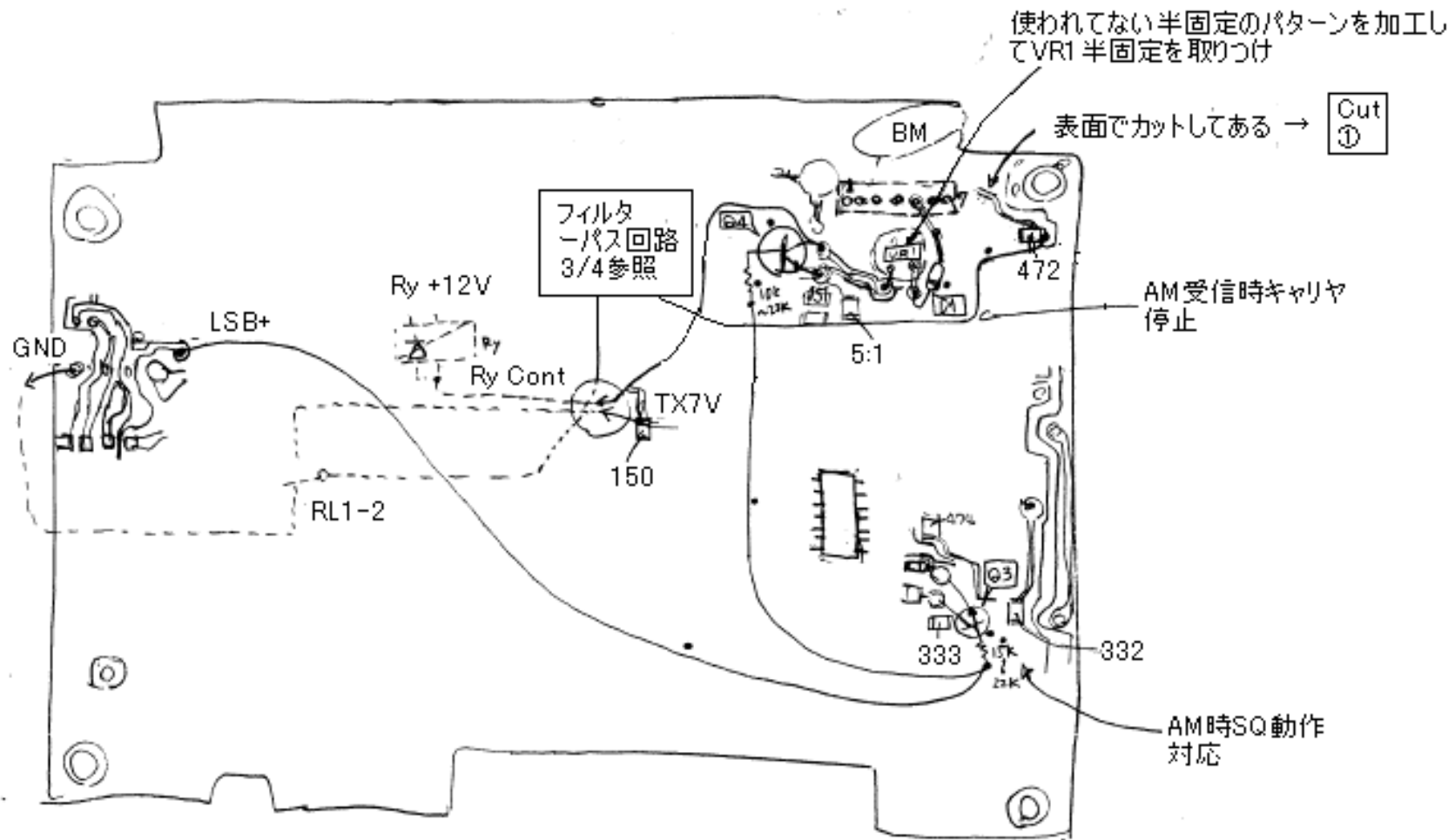
MAIN UNIT 裏側実装状況
