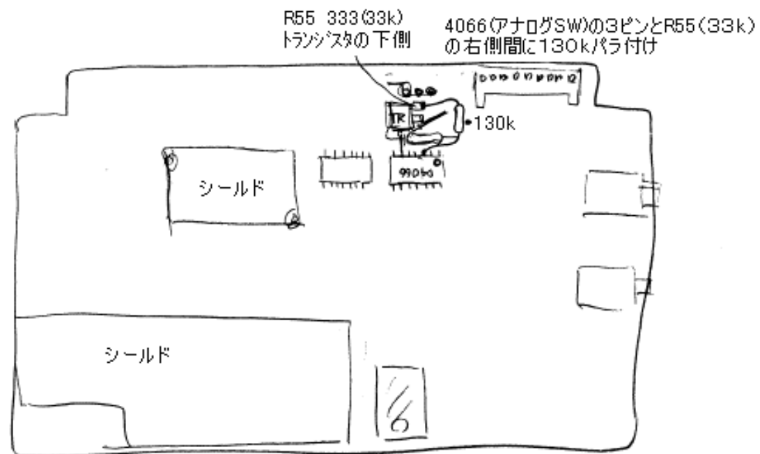
PLL/PA基板実装状況
